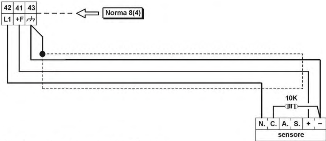
Figura 8 Collegamento di un sensore con linea bilanciata.
