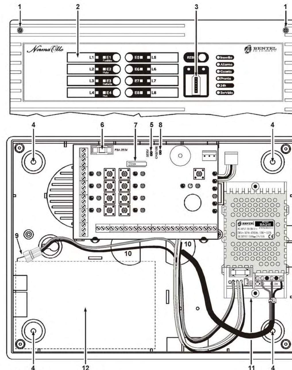
Figura 2 Parti della centrale versione NormaOtto/K
