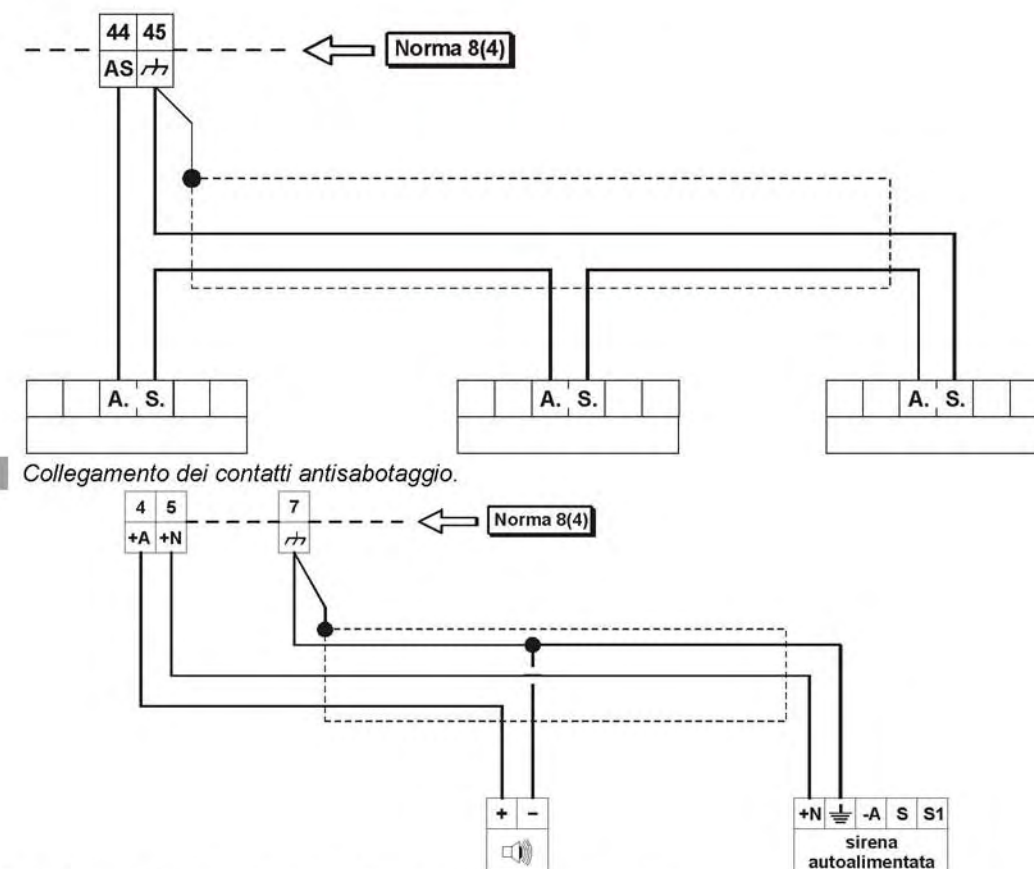
Figura 13 Collegamento con una sirena autoalimentata ed una per interno.
