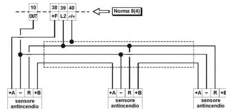
Figura 11 Esempio di collegamento di sensori antincendio.
