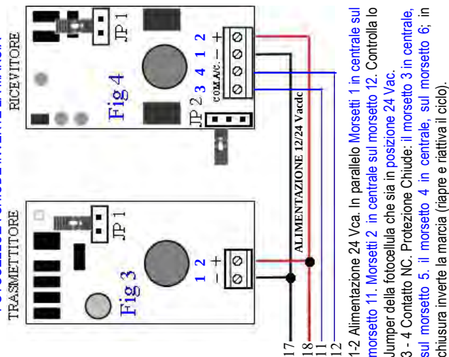
FOTOCELLULA CHIUDI INVERTE LA MARCIA
