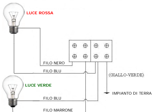
SCHEMA DI COLLEGAMENTO LAMPADE
