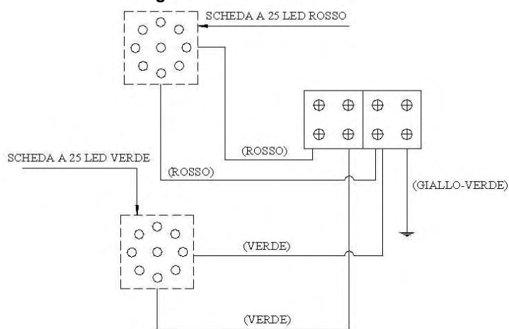
Shema di collegamento delle schede a 25 Led 24 V
